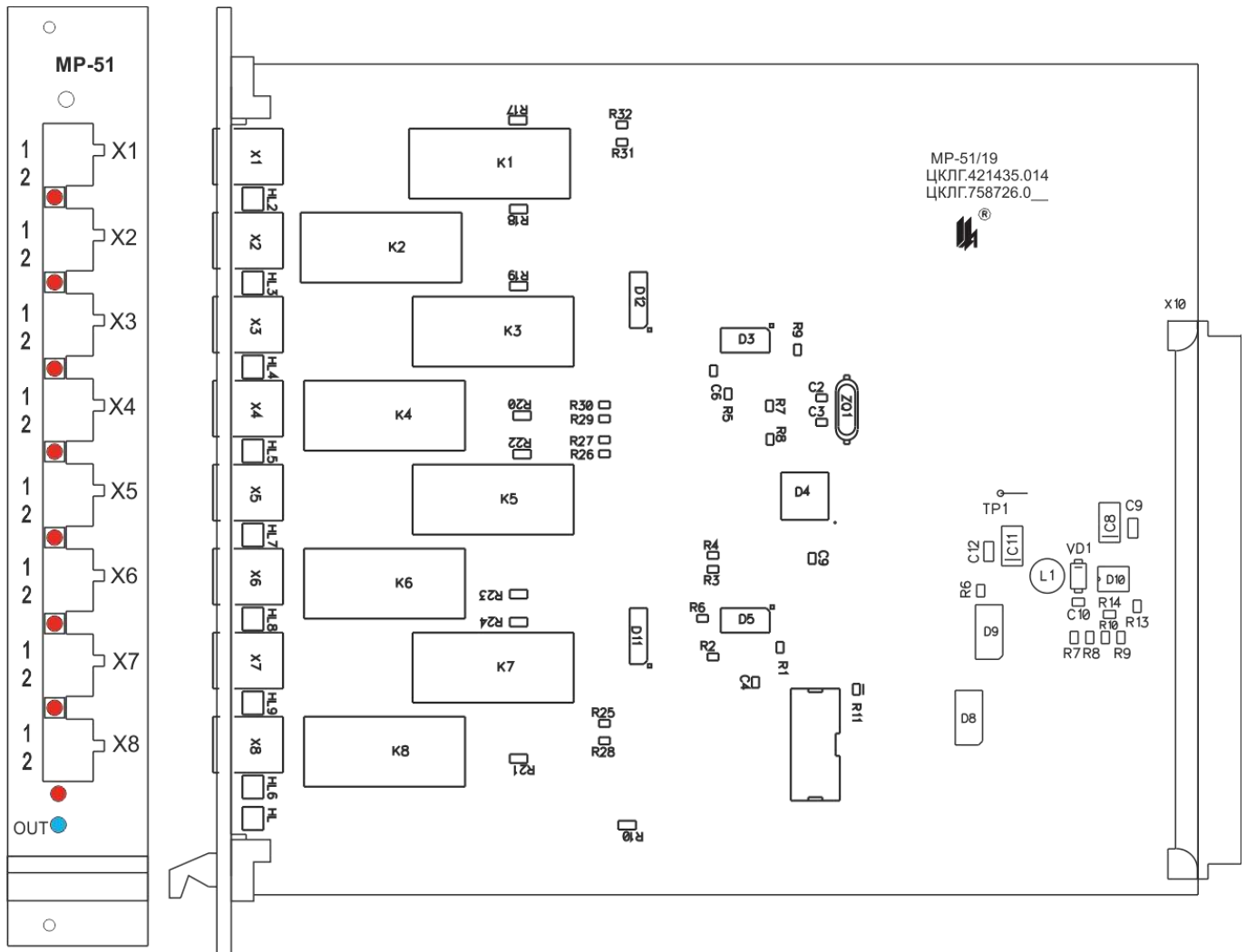
Рисунок 4.14 – Плата модуля реле MP-51/19
