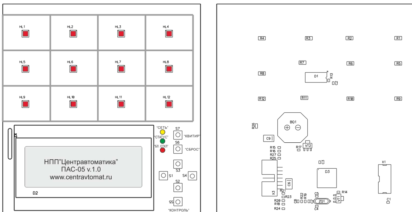
Рисунок 4.1 – Плата модуля индикации МДИ5-12
