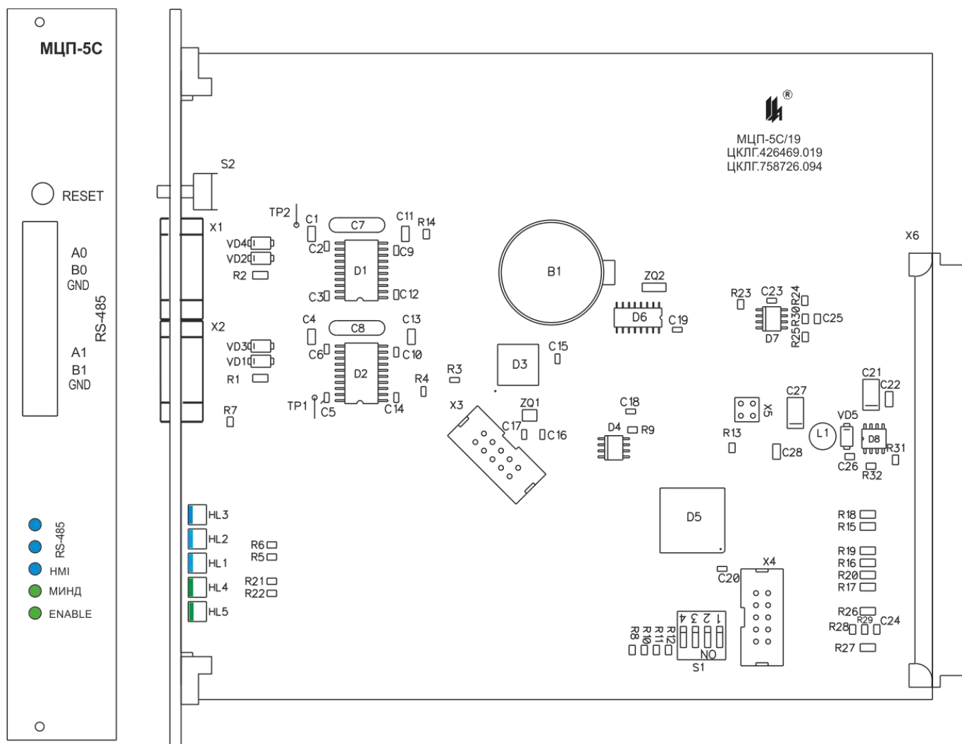
Рисунок 4.6 – Плата модуля центрального процессора МЦП-5С/19
