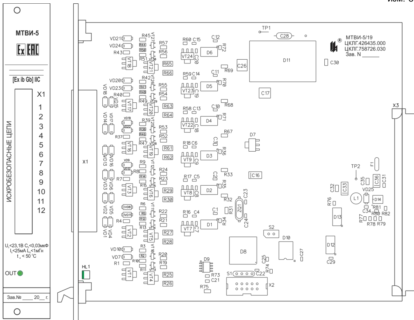
Рисунок 4.21 – Плата модуля токового вывода искробезопасного МТВИ-5/19
