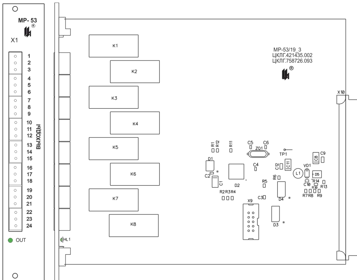
Рисунок 4.13 – Плата модуля реле MP-53/19
