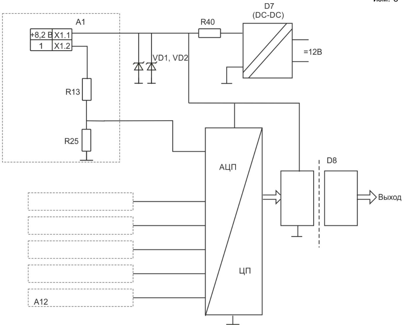
Рисунок 5.2 – Схема узлов, обеспечивающих искробезопасность цепей МВДС-9
