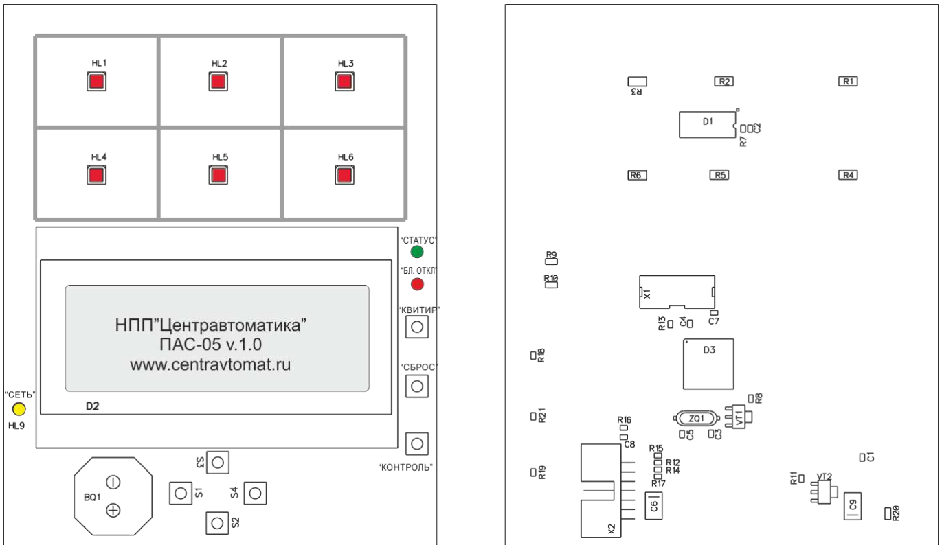
Рисунок 4.2 – Плата модуля индикации МДИ5-6
