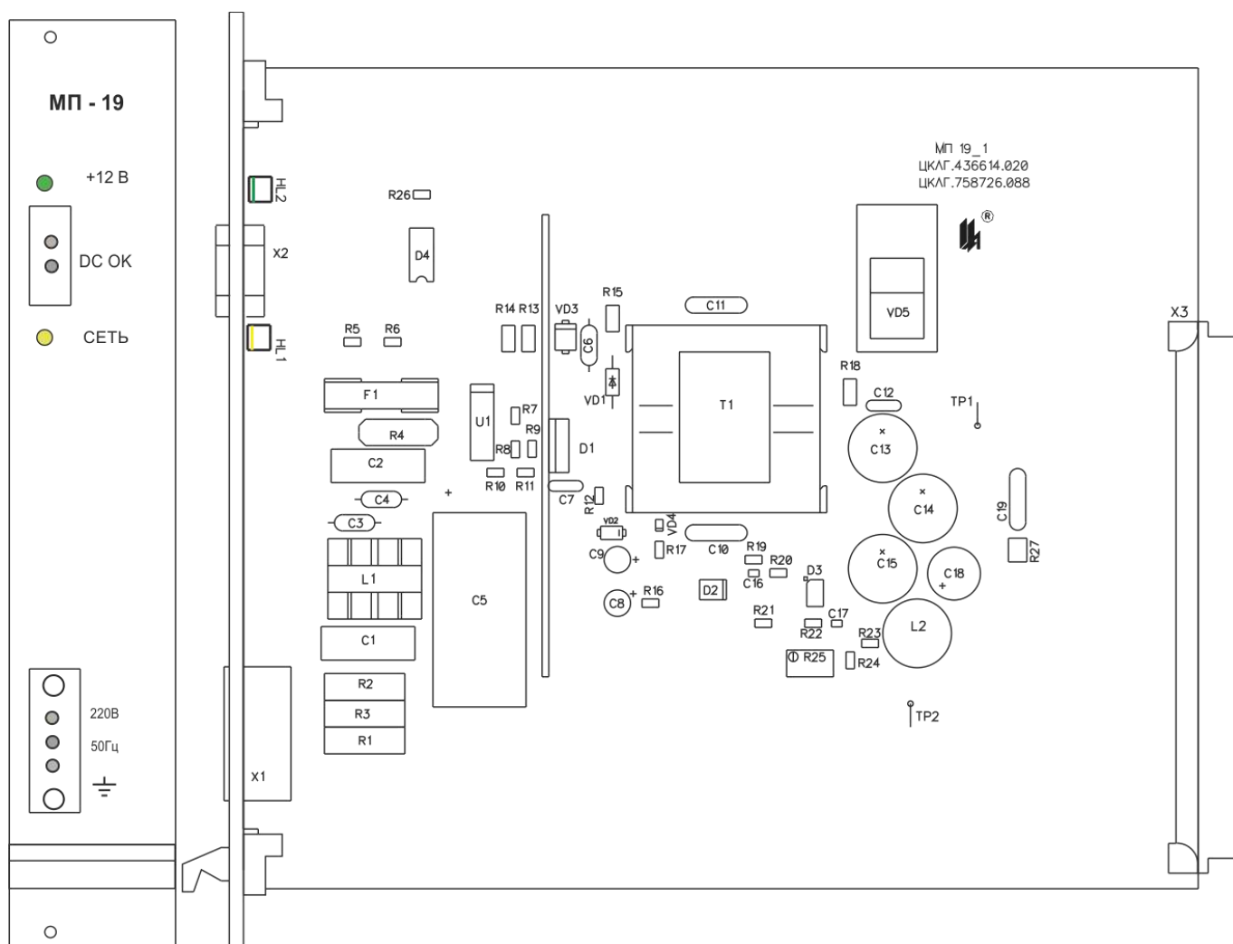
Рисунок 4.10 – Плата модуля питания МП-19
