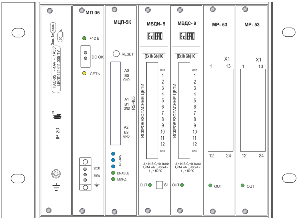
Рисунок 1.2 – Внешний вид ПАС-05-4А (со стороны лицевой панели и со стороны установки модулей)
