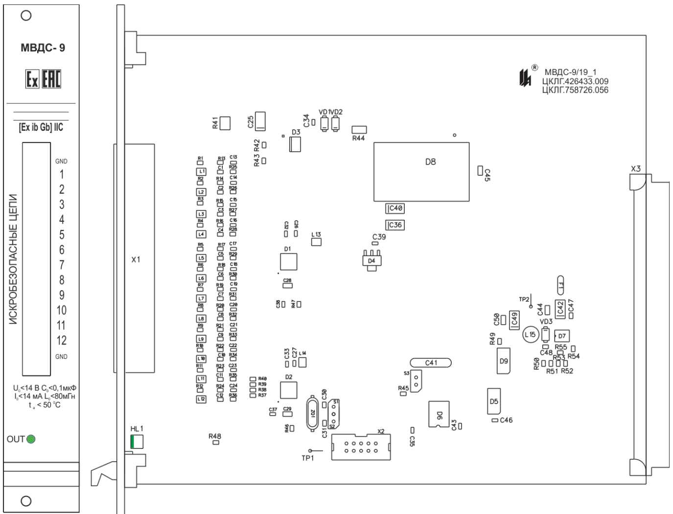
Рисунок 4.12 - Внешний вид платы модуля ввода МВДС-9/19
