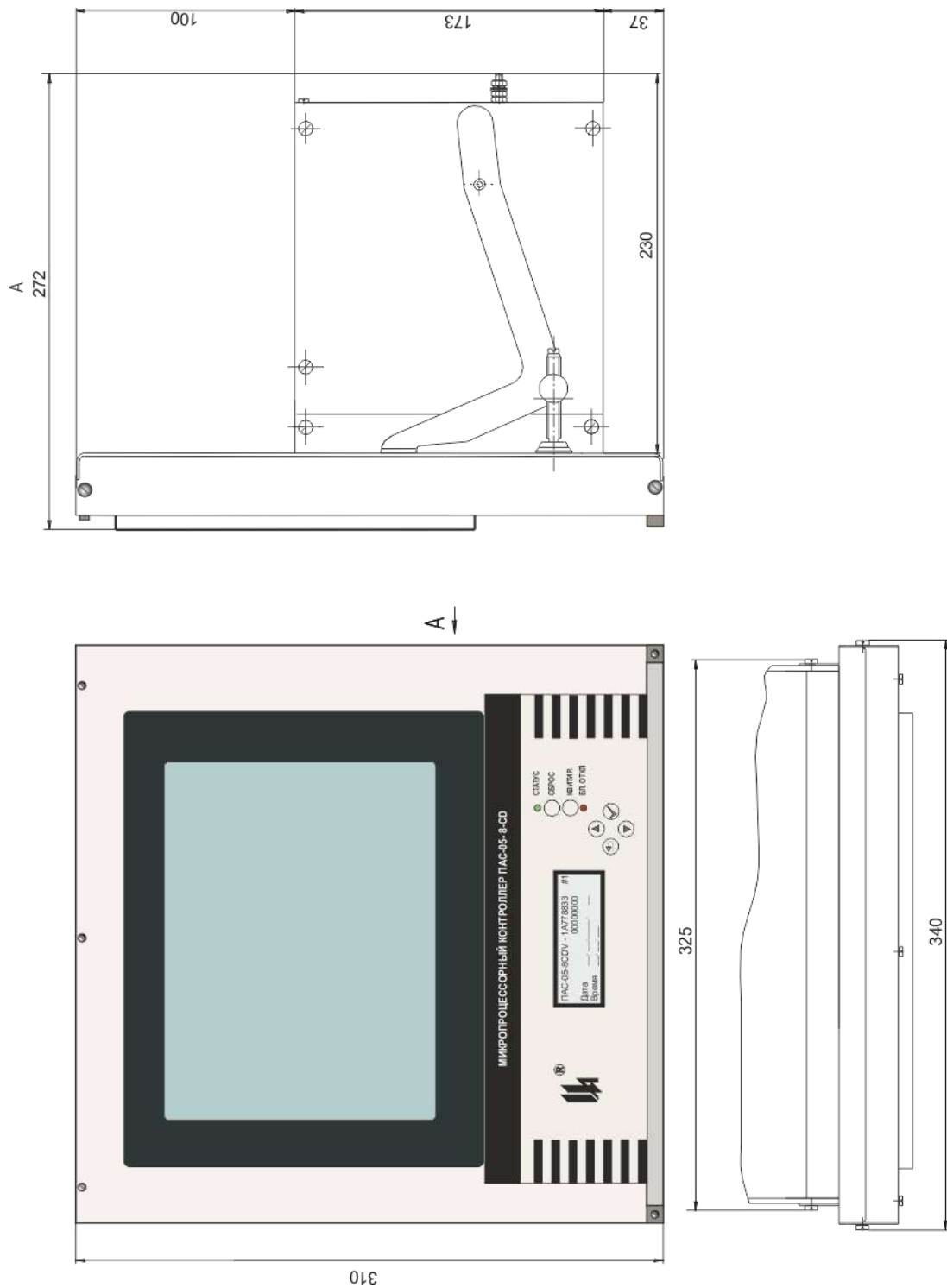
Рисунок 1.5 – Внешний вид ПАС-05-8CD, ПАС-05-7DR и ПАС-05-8CDU
