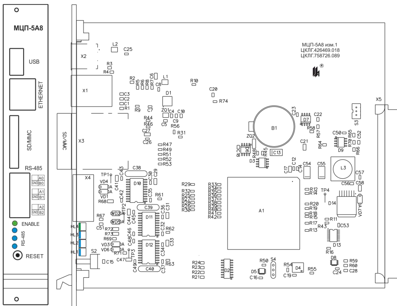
Рисунок 4.8 – Плата модуля центрального процессора МЦП-5A8
