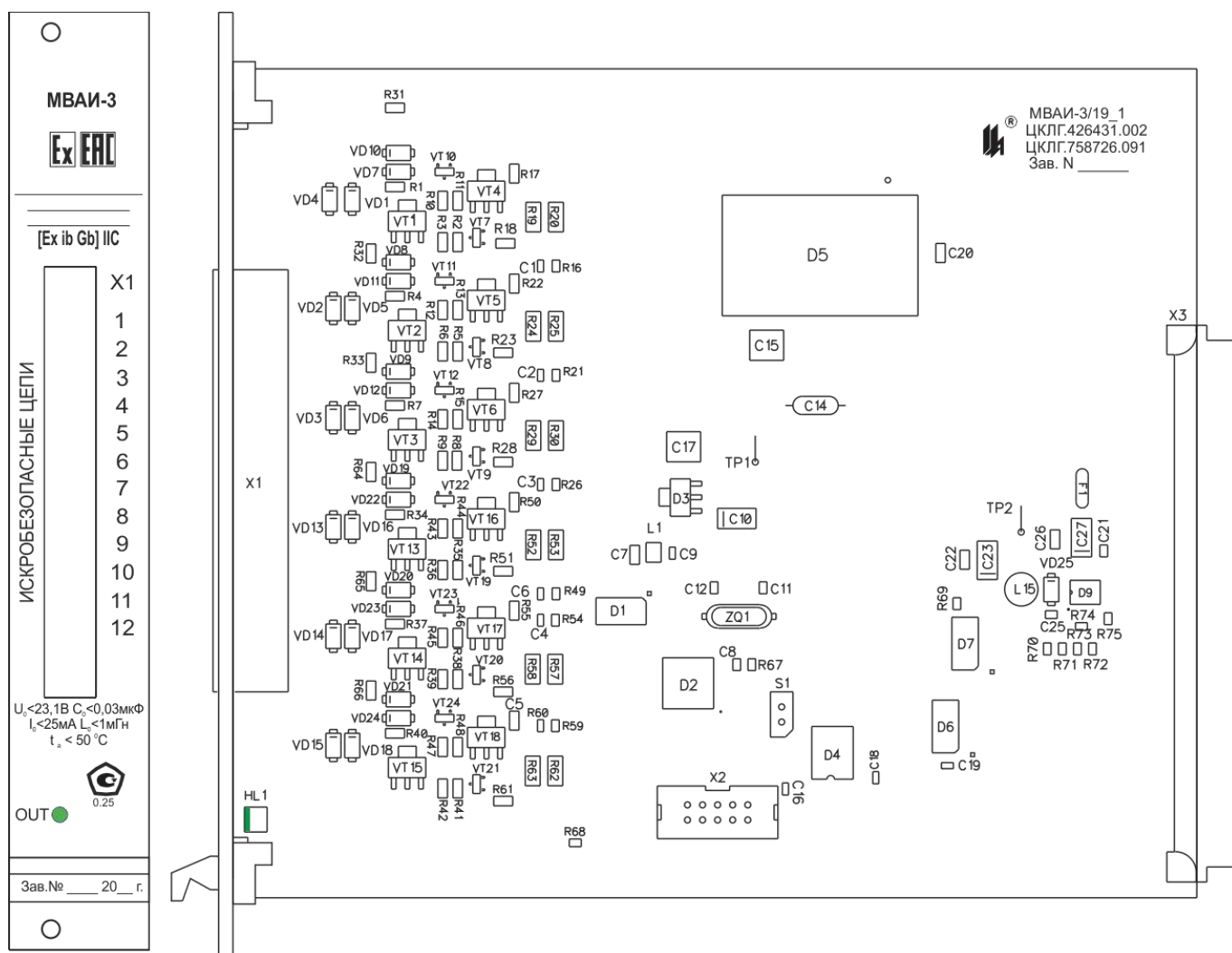
Рисунок 4.15 – Плата модуля ввода аналоговой информации МВАИ-3
