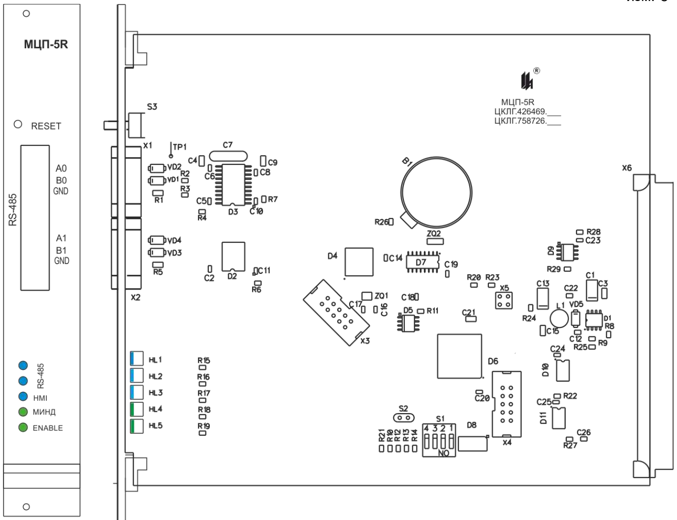
Рисунок 4.7 – Плата модуля центрального процессора МЦП-5R/19
