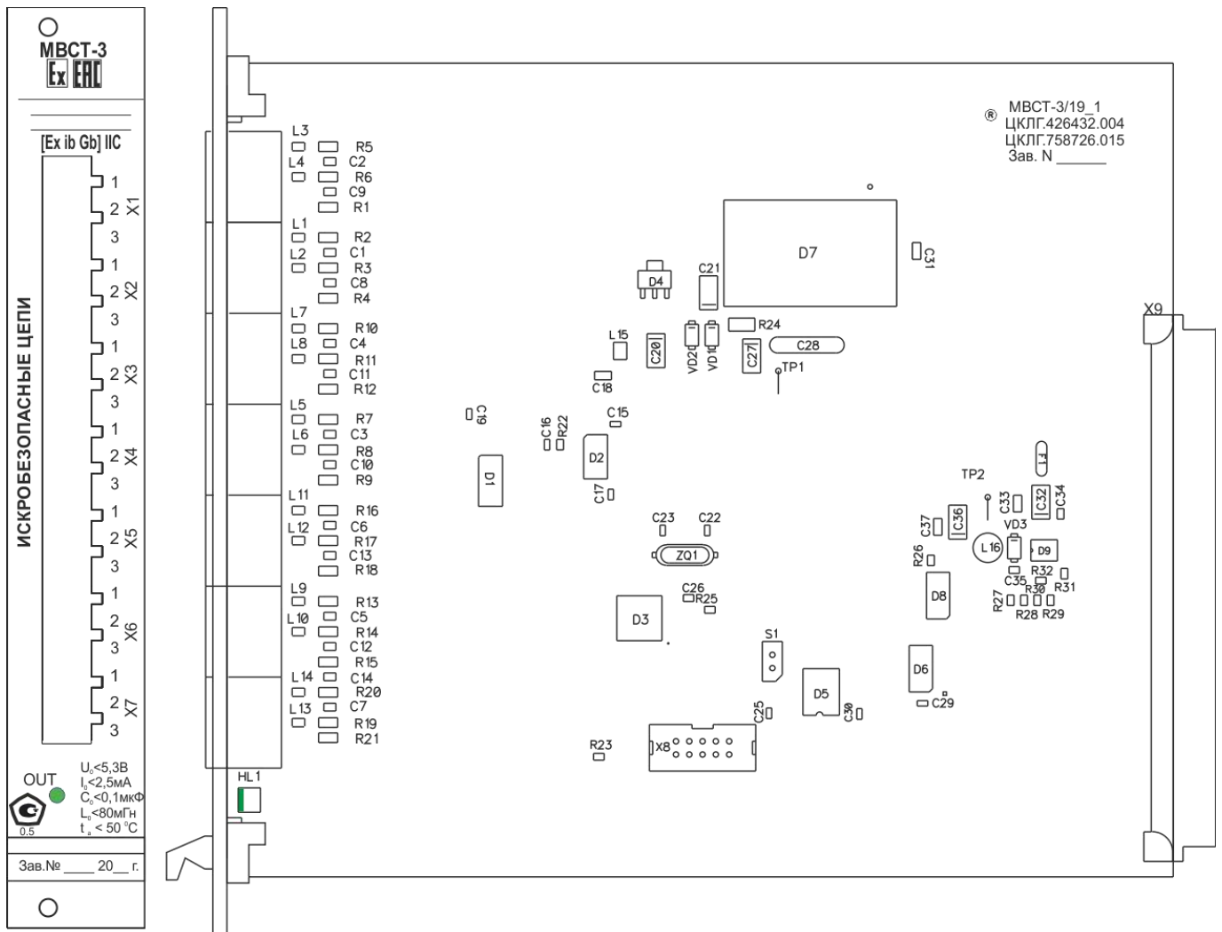
Рисунок 4.17 – Плата модуля ввода сигналов термopеобразователей MBCT-3
