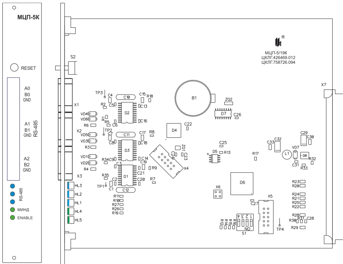
Рисунок 4.5 – Плата модуля центрального процессора МЦП-5К/19
