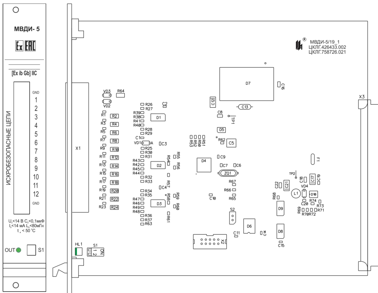
Рисунок 4.11 – Плата модуля ввода дискретной информации МВДИ-5
