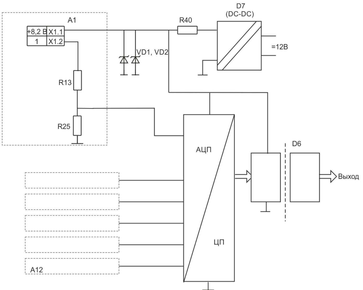
Рисунок 5.1 – Схема узлов, обеспечивающих искробезопасность цепей МВДИ-5
