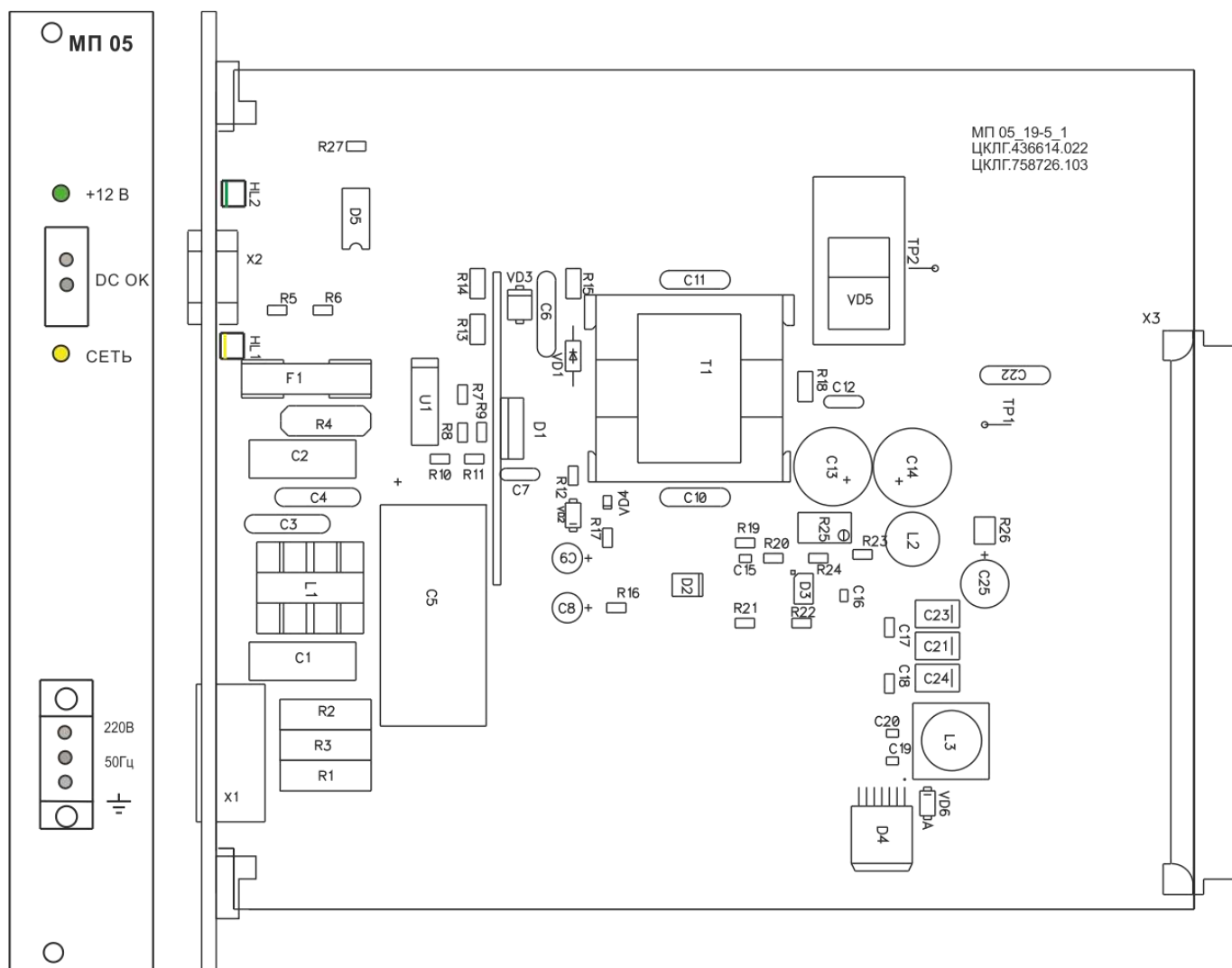
Рисунок 4.9 – Плата модуля питания МП-05/19
